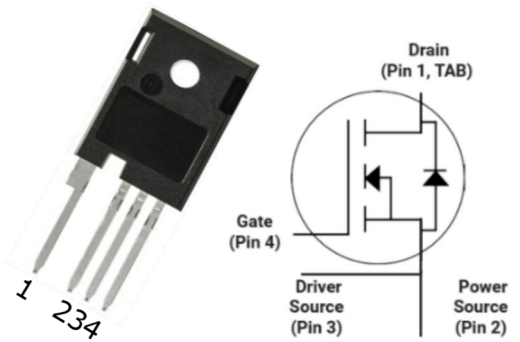
TO-247-4L
