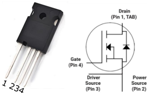
TO-247-4L
