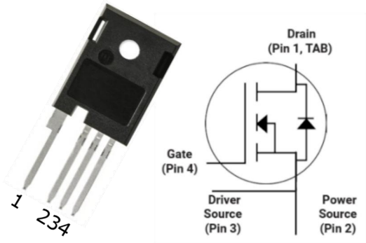
TO-247-4L
