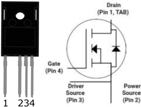
TO-247-4L
