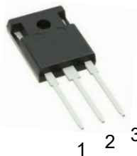
TO-247-3L
