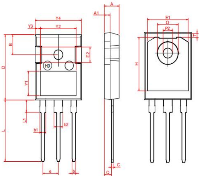
TO-247-3L-B
