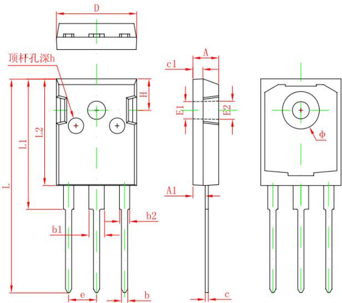
TO-247-3L-A
