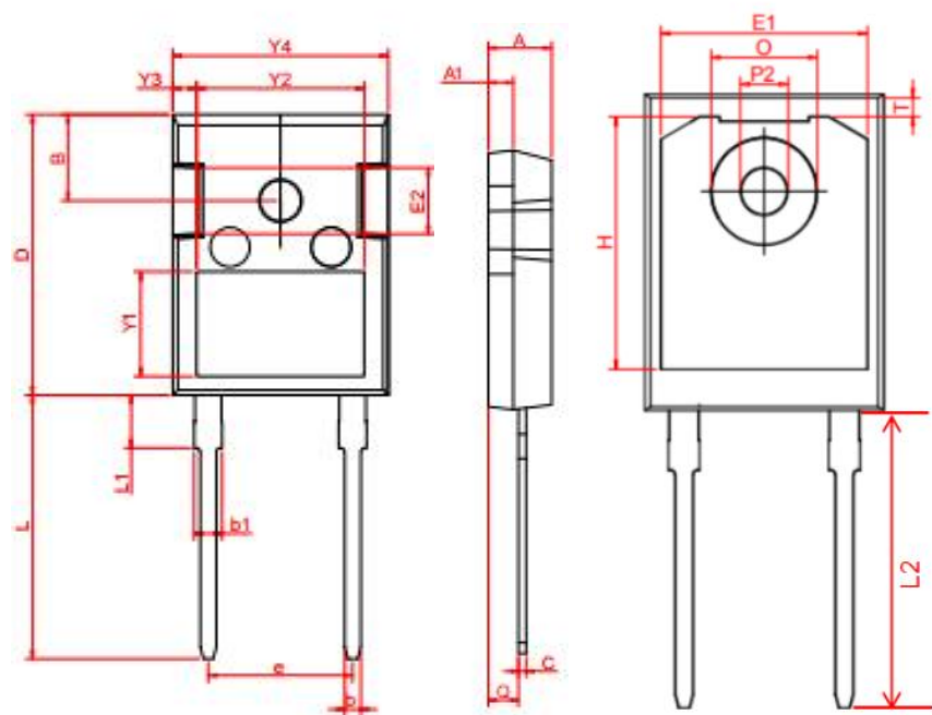
TO-247-2L-B
