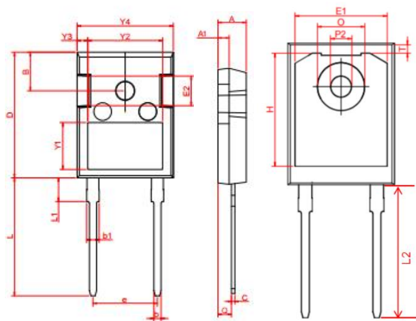
TO-247-2L-B
