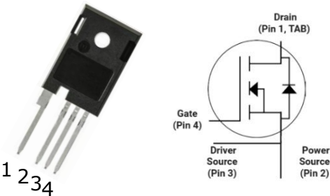
TO-247-4L
