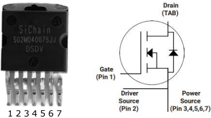
TO-263-7L
