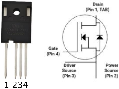
TO-247-4L
