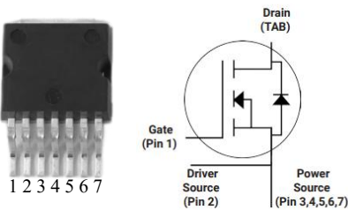
TO-263-7L
